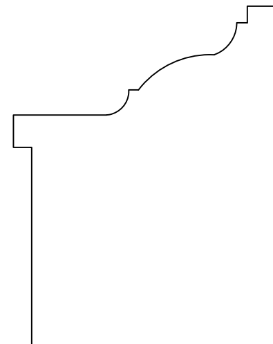
PC2002 2-9/16" x 2"
