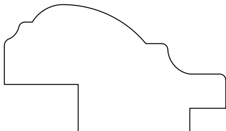
PC2372 1-3/8" x 2-3/8"
